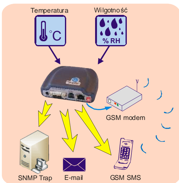
Rys.1 Schemat działania Posejdona 3265
